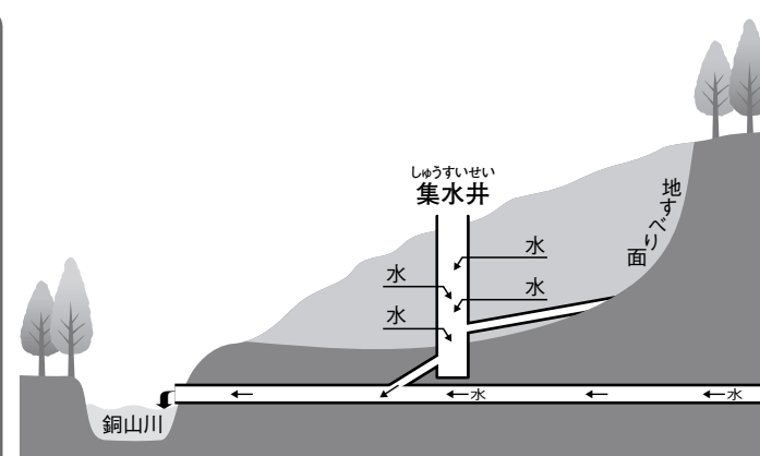
▲集水井に地下水が集まる様子
