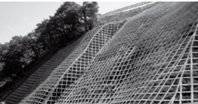
寒風田法枠工（平成24年度施工）
