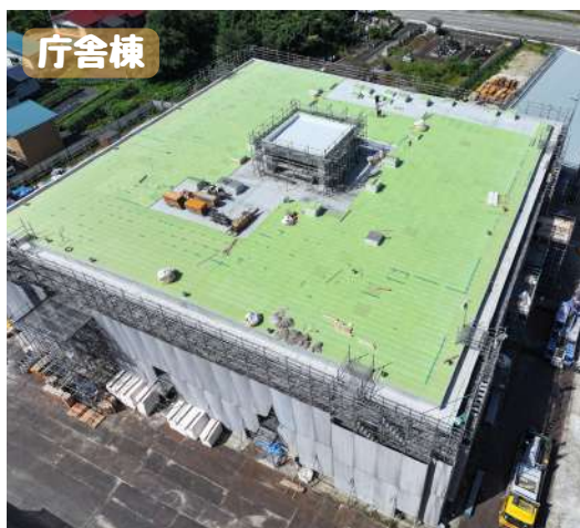
庁舎棟
